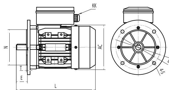
B5
