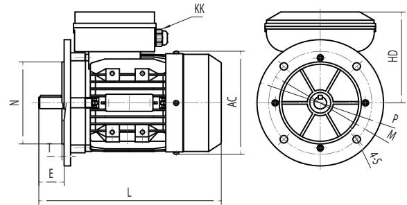
B5
