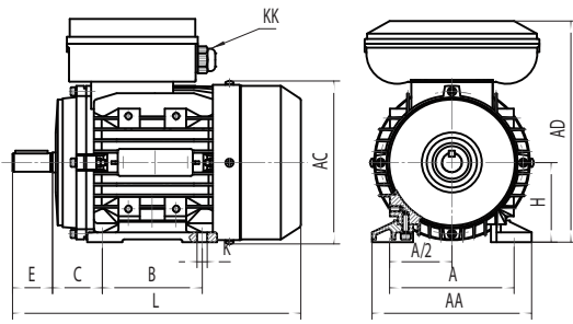
B3
