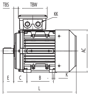
B3
