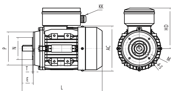
B14
