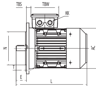
B5
